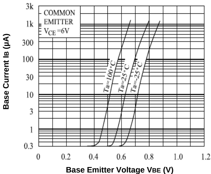
Fig.5- I_B - V_{BE}
