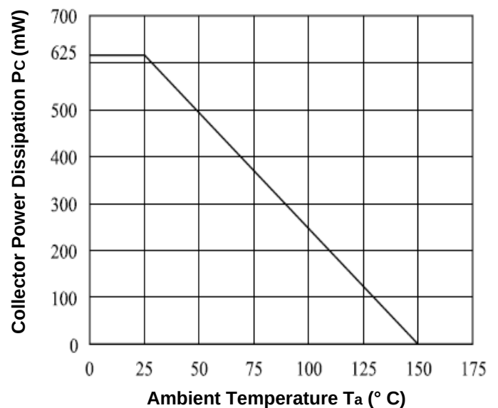
Fig.6- P_C - T_a
