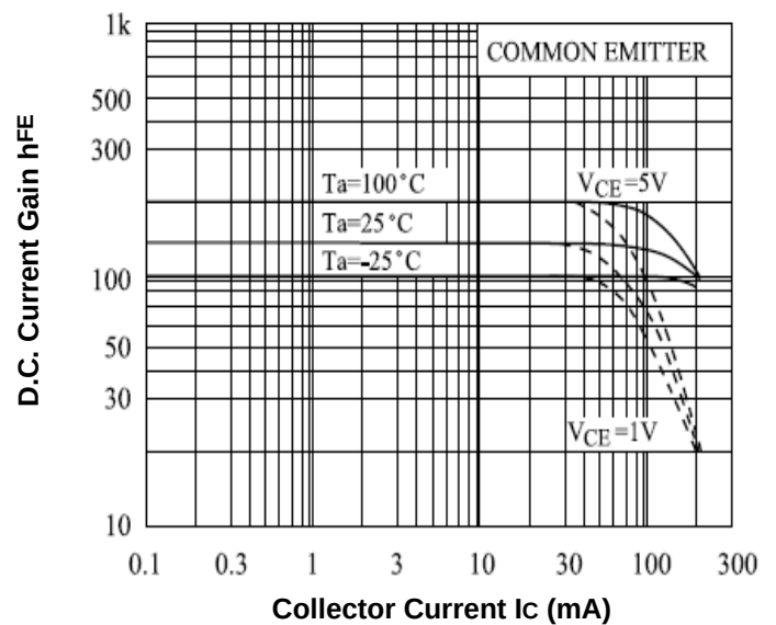
Fig.2- h_{FE} - I_C
