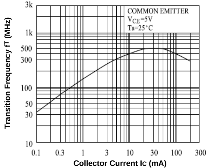
Fig.4- f_T - I_C
