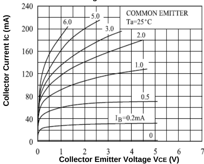
Fig.1- I_C - V_{CE}
